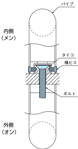
1 両面用(タイプA)
