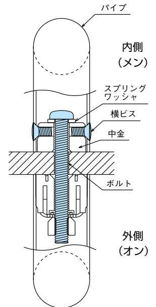
4 両面用(タイプB)
